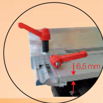
BLOCCAGGIO SQUADRETTA rigidissimo e regolabile STAINLESS STEEL BRACKET LOCK extra rigid and adjustable
