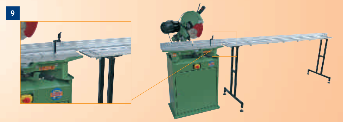
- RULLIERA COMPLETA DI PIEDI (LUNGHEZZA A RICHIESTA MIN. MT 1,00) - LOADING ROLLER WITH SUPPORT (LENGHT ON REQUEST MIN. MT 1,00)
