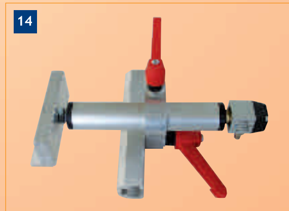
- COPPIA MORSE ORIZZONTALI PNEUMATICHE PER CORNICI - COUPLE PNEUMATIC HORIZONTAL CLAMP FOR FRAME
